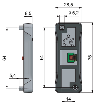
Striker plate
