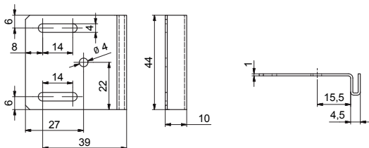
Striker plate
