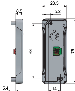
RFID reader L043-A02
