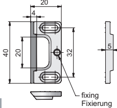
Striker plate
