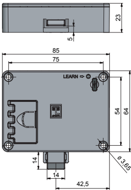
RFID reader L043-A01
